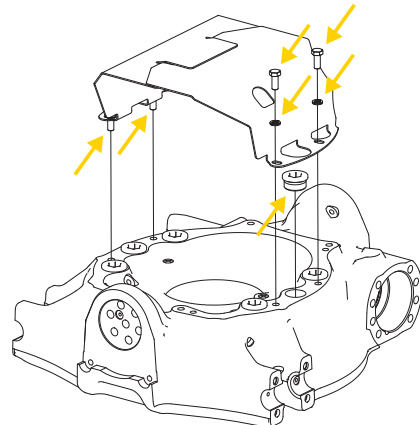
Afbeelding14. Demonstreer de beschermkap.
